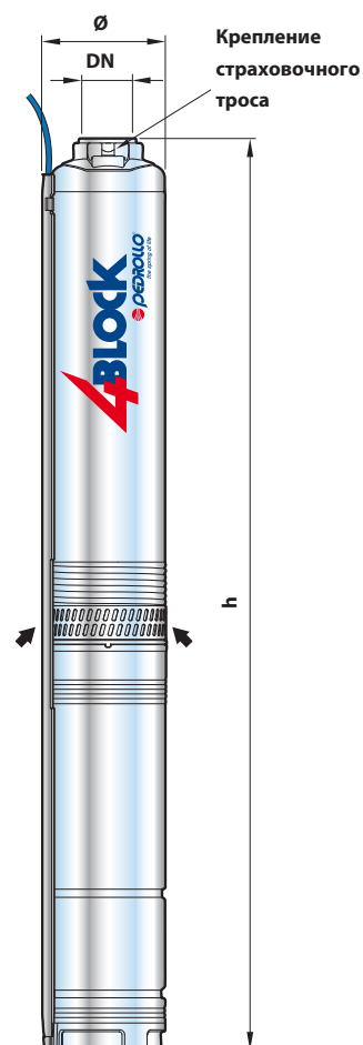
Стандартная установка
