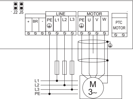
Fig.7 Size E
