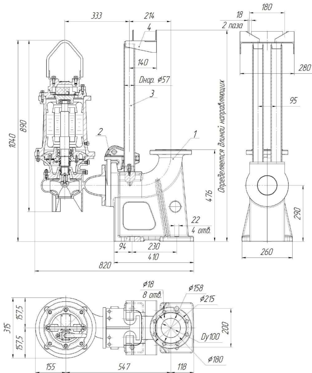
Рис. 91 Общий вид и габаритные размеры электронасоса "Иртыш" ПФ2 100/150 – 7,5/2– 106 с опускным устройством
