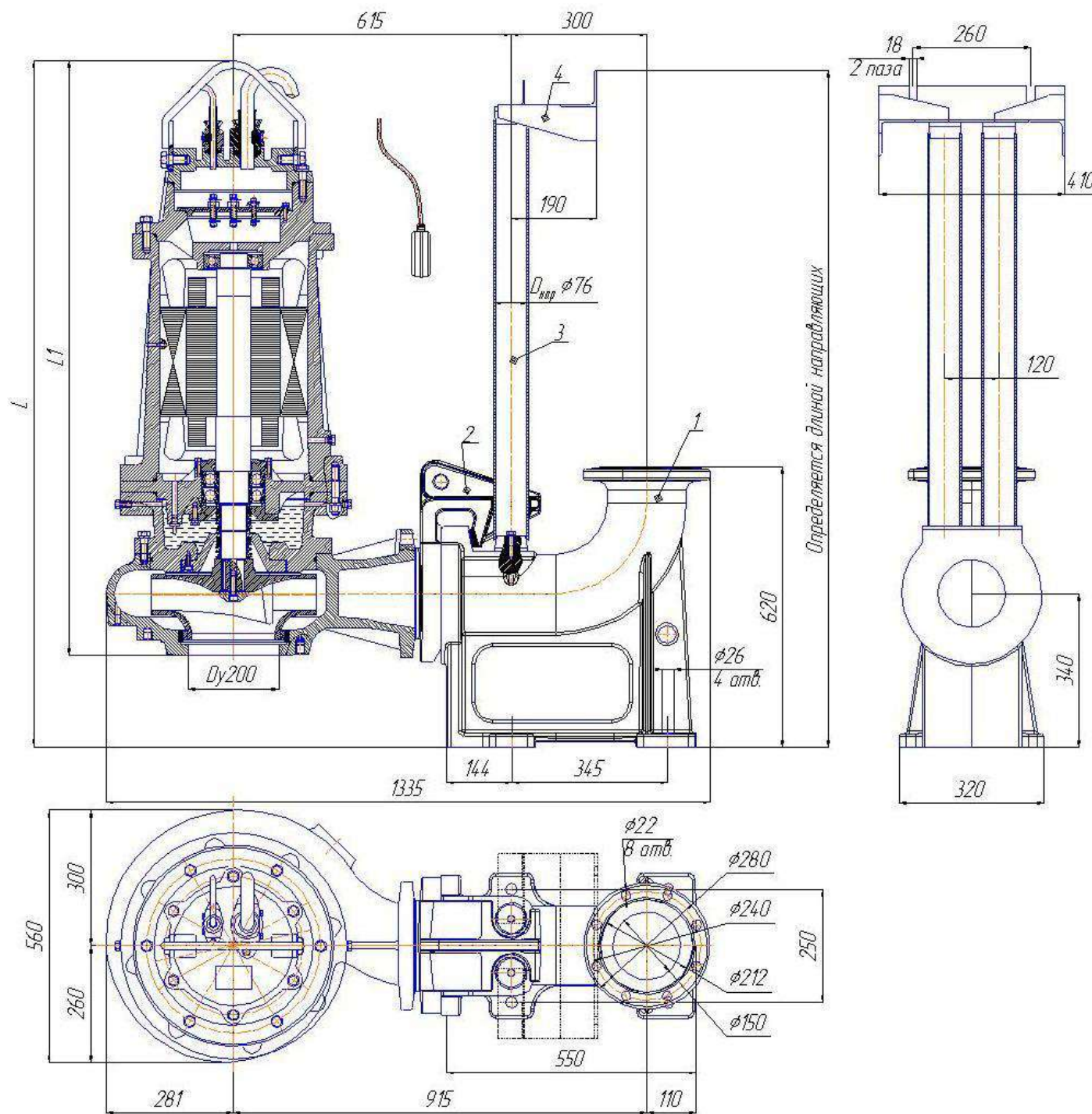
Рис. 104 Общий вид и габаритные размеры электронасоса "Иртыш" ПФ2 150/315 – 22/6– 106; ПФ2 150/315 – 37/4– 106; ПФ2 150/315 – 45/4– 106; ПФ2 150/315 – 55/4– 106 с опускающим устройством.
