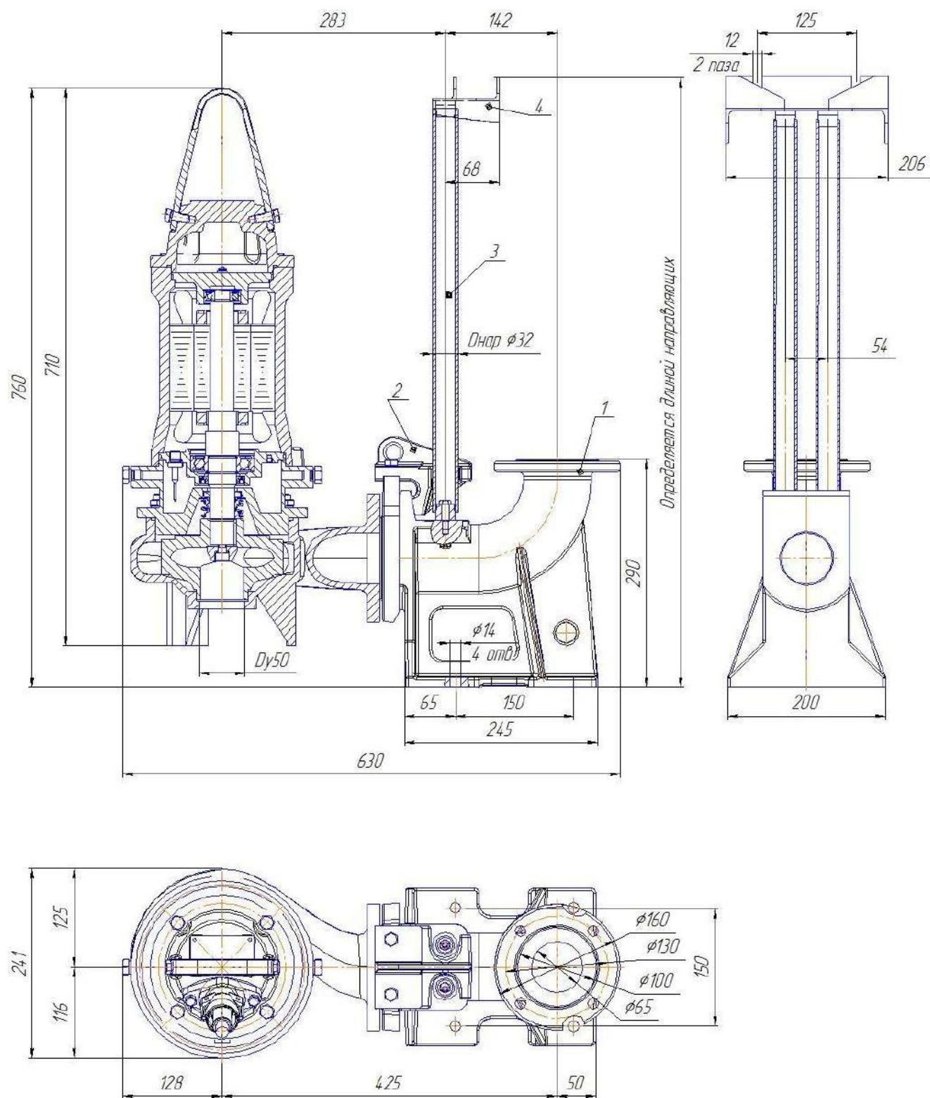
Рис. 74 Общий вид и габаритные размеры электронасоса "Иртыш" ПФ2 65/155 – 3/2 -106 с опускным устройством
