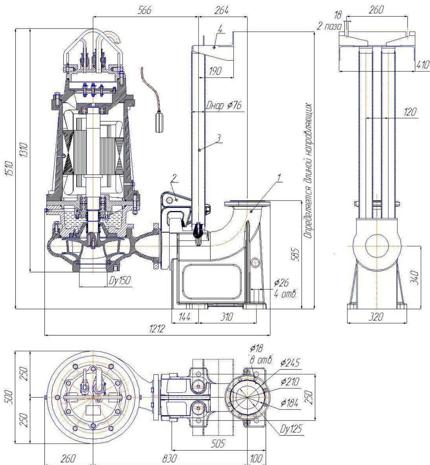
Рис. 97 Общий вид и габаритные размеры электронасоса "Иртыш" ПФ2 125/315 – 37/4 – 106 с опускающим устройством.
