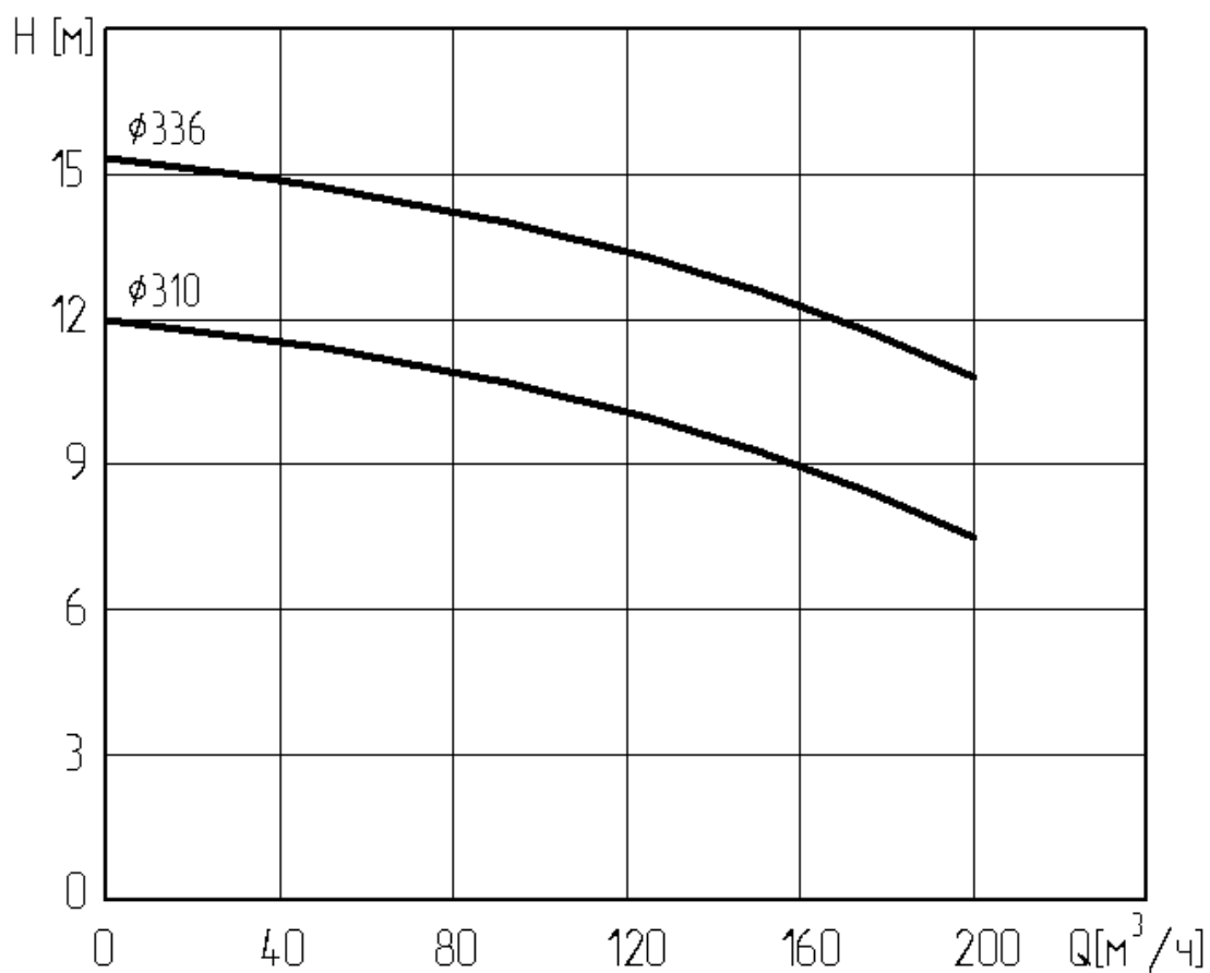
Рис. 9 Рабочие характеристики насоса «Иртыш»:
