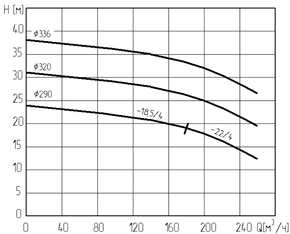
Рис. 10 Рабочие характеристики насоса «Иртыш»:
